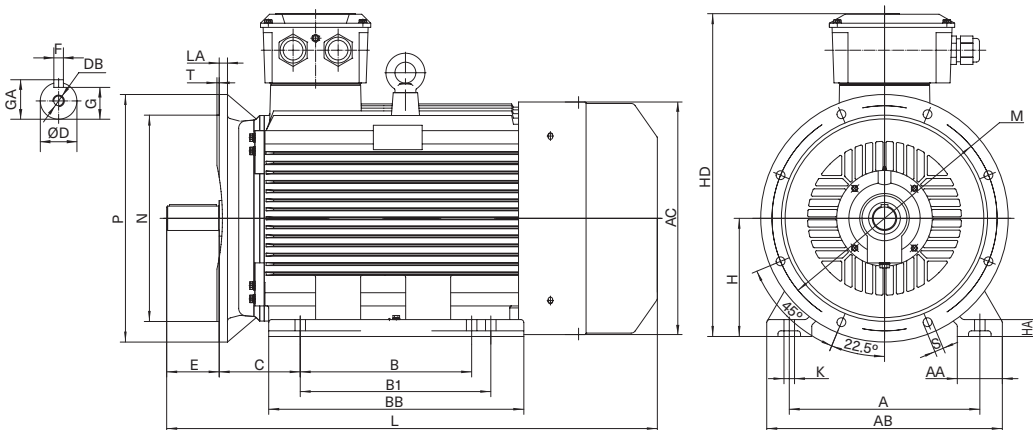
底脚和凸缘安装电机 IMB35、IMV15、IMV36 Foot- and big flange-mounted motor IMB35、IMV15、IMV36
